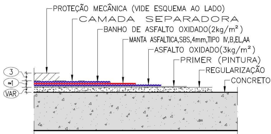
Figura 1 - Imagem ilustrativa das camadas a serem executadas.
